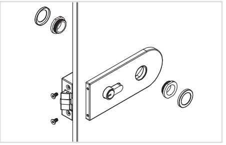
Utilice pieza guía para apretar roseta Use plastic driver to tighten rose
